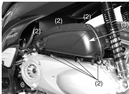
(2) Tornillos
