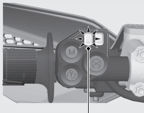
Testigo (ámbar) de avería (MIL) de la PGM-FI/testigo (azul) de modo del motor
