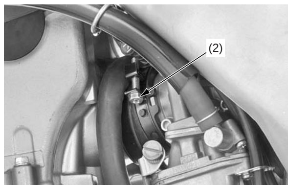
(2) tornillo de la banda del aislador
