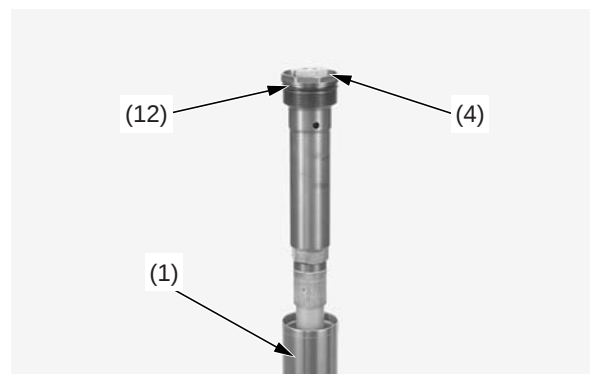
(1) tubo exterior (4) conjunto del amortiguador de la horquilla (12) Junta tórica
