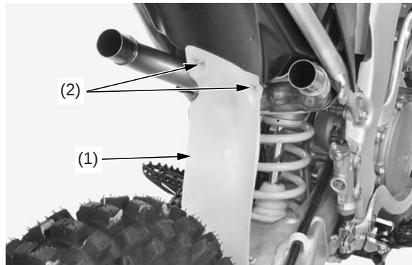
(1) parafangos (2) tornillos
