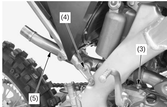
(3) Perno de la abrazadera del tubo de unión (4) perno de montaje del tubo de unión de escape (5) tubo de unión de escape
