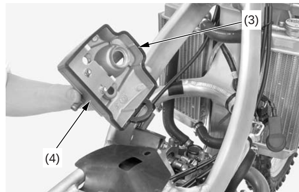
(3) empaquetadura de la cubierta de la culata de cilindros (4) cubierta de la culata de cilindros
