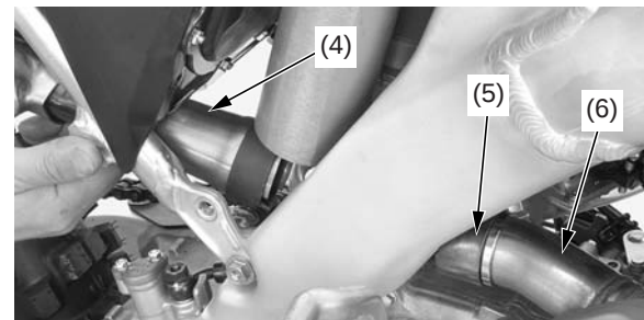
(4) tubo de unión de escape (5) empaquetadura (6) tubo de escape
