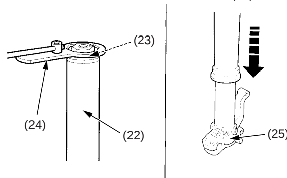
(22) tubo exterior (23) amortiguador de la horquilla (24) llave de contratuerzas (25) corredera, extremo inferior
