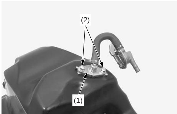
(1) junta de combustible (2) pernos
