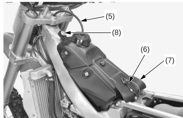
(5) tubo del respiradero (6) banda del depósito de combustible (7) goma de la cubierta del filtro de aire (8) perno del depósito de combustible
