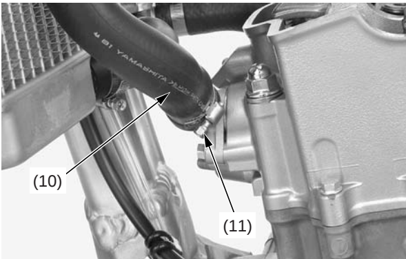
(10) manguera del radiador (11) abrazadera de la manguera del radiador
