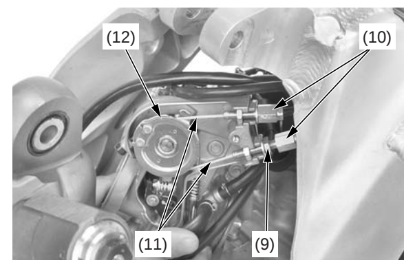
(9) contratuerca (10) ajustadores (11) cables del acelerador (12) tambor del acelerador
