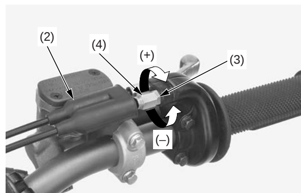
(2) cubierta contra el polvo (3) contratuerca (4) ajustador superior (+) incrementar (-) reducir
