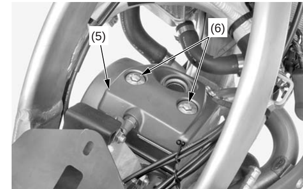
(5) cubierta de la culata de cilindros (6) pernos de la cubierta de la culata de cilindros
