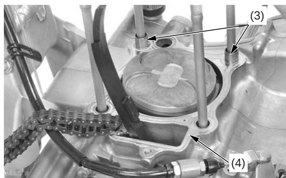
(3) pasadores cónicos (4) empaquetadura del cilindro
