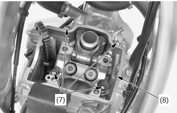
(7) tuercas/arandelas de la culata de cilindros (8) culata de cilindros
