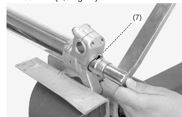
(7) junta tórica del perno central
