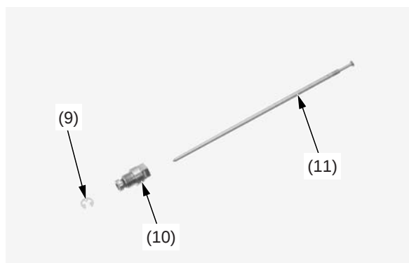
(9) retenedor (10) soporte de la aguja del surtidor (11) aguja del surtidor
