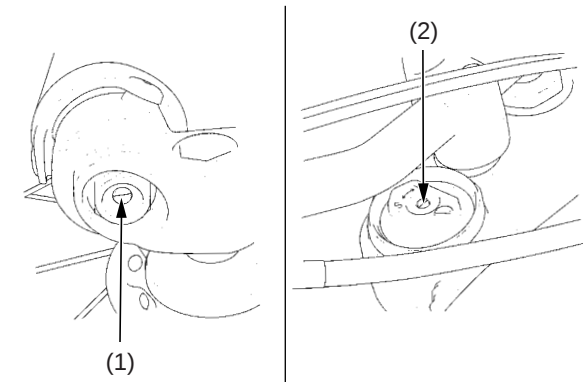
(1) tornillo del ajustador de la amortiguación de expansión (2) tornillo del ajustador de la amortiguación de compresión
