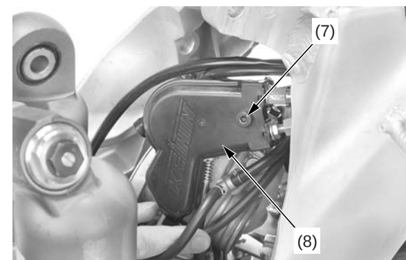
(7) perno de la cubierta del tambor del acelerador (8) cubierta del tambor del acelerador
