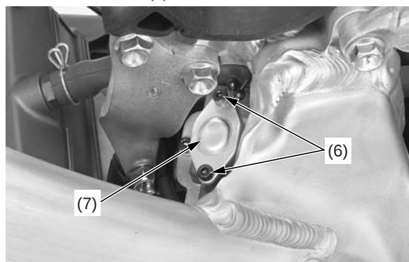
(6) pernos superiores del carburador (7) parte superior del carburador
