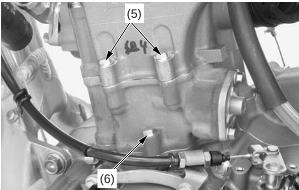
(5) pernos de la culata de cilindros (6) perno del cilindro
