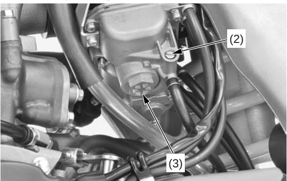
(2) tornillo de drenaje (3) tapón de la taza del flotador
