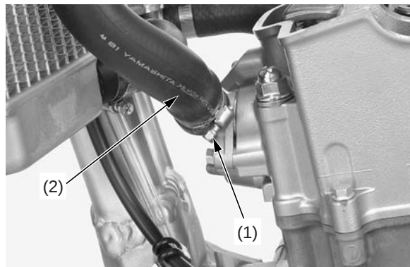
(1) abrazadera de la manguera de agua (2) manguera de agua
