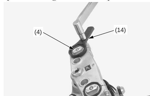
(4) conjunto del amortiguador de la horquilla (14) llave de contratuerzas
