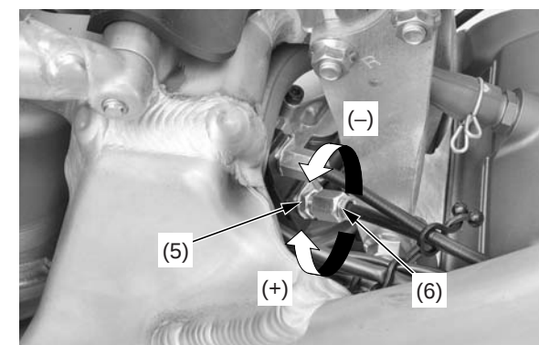
(5) contratuerca (6) ajustador inferior (+) incrementar (-) reducir
