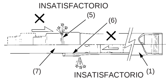
(1) tubo exterior (5) sello contra el polvo (6) buje de la guía (7) corredera
