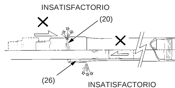
(20) sello contra el polvo de la horquilla (26) buje de la guía
