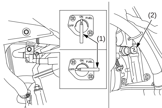
(1) válvula del combustible (2) perilla del estrangulador
