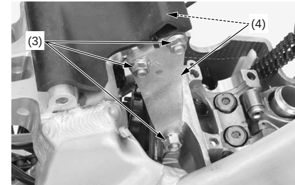
(3) pernos/tuercas del soporte del motor (4) placas del soporte del motor
