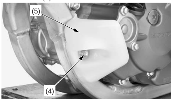
(4) perno del protector izquierdo del motor (5) protector izquierdo del motor
