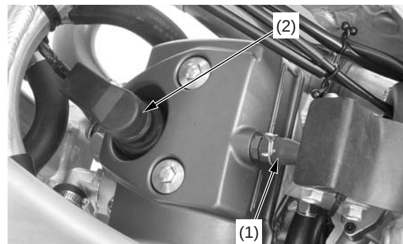
(1) tubo del respiradero (2) bobina de encendido directo
