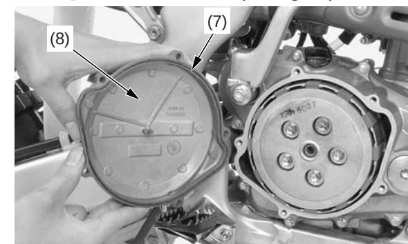
(7) junta tórica (8) cubierta del embrague
