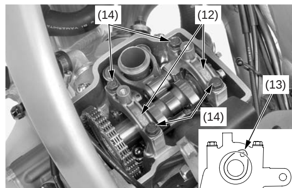
(12) soportes del árbol de levas (13) lóbulos de las levas de admisión (14) pernos de los soportes del árbol de levas
