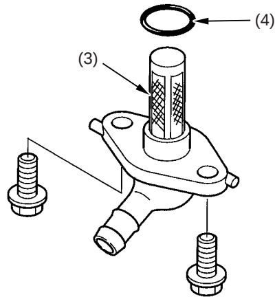
(3) filtro de combustible (4) Junta tórica
