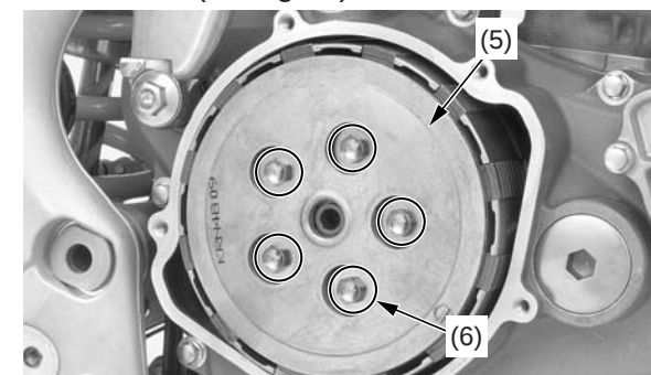
(5) placa de presión del embrague (6) pernos de los resortes del embrague/resortes del embrague
