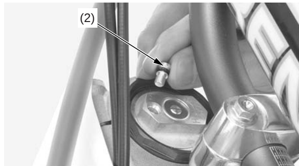
(2) tornillos de liberación de la presión
