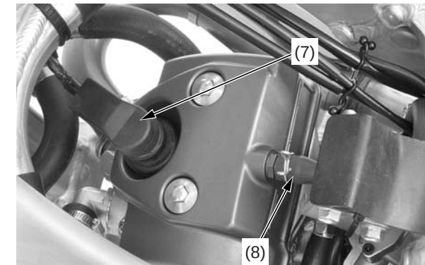
(7) bobina de encendido directo (8) tubo del respiradero
