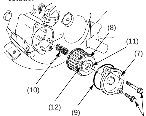
(6) pernos de la cubierta del filtro de aceite (7) cubierta del filtro de aceite (8) filtro de aceite (9) junta tórica de la cubierta del filtro de aceite (10) resorte (11) sello de goma (12) marca "OUT-SIDE"
