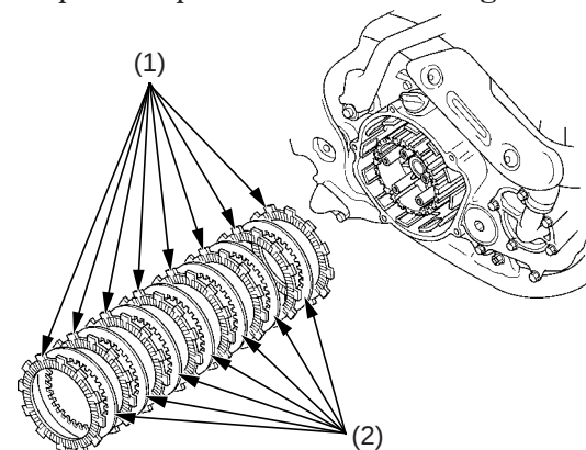
(1) discos del embrague (2) placas del embrague
