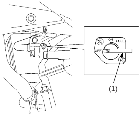
(1) válvula del combustible
