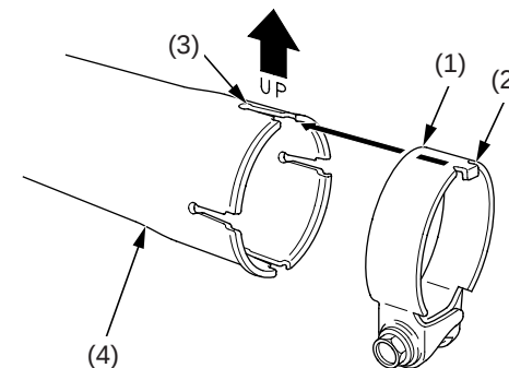
(1) abrazadera del tubo de unión (2) lengüeta (3) corte (4) tubo de unión de escape
