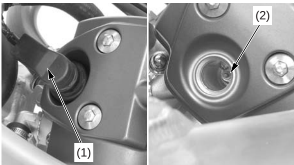
(1) bobina de encendido directo (2) bujía
