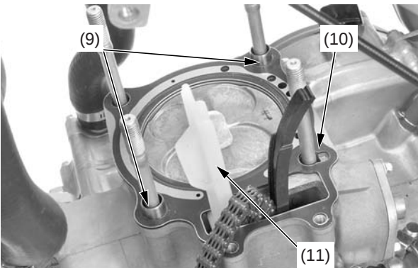
(9) pasadores cónicos (10) empaquetadura de la culata de cilindros (11) guía de la cadena de levas
