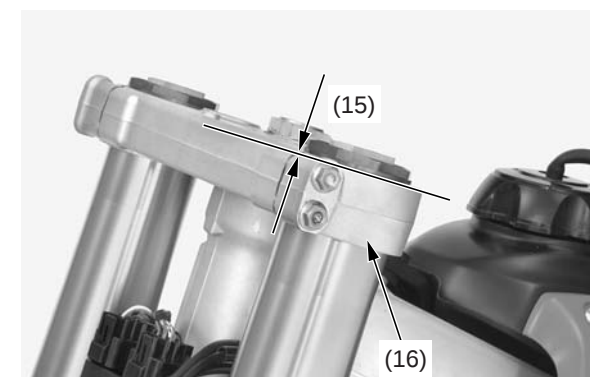
(15) alinear (16) abrazadera de la horquilla superior
