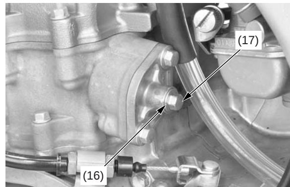
(16) arandela de sellado (17) perno de la cubierta del alzador del tensor de la cadena de levas
