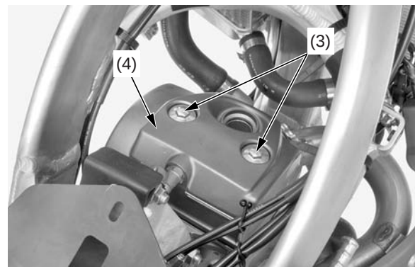
(3) pernos de la cubierta de la culata de cilindros (4) cubierta de la culata de cilindros
