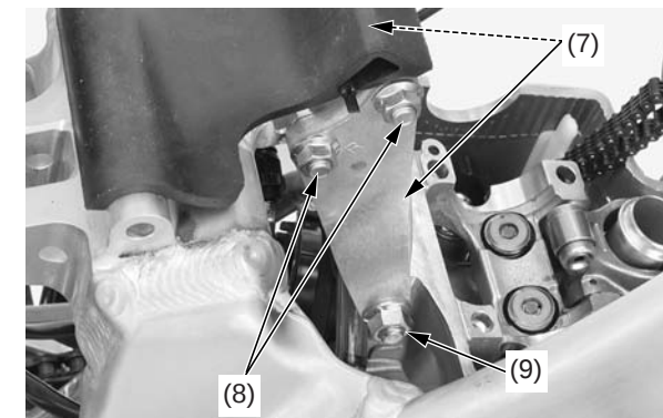
(7) placas del soporte del motor (8) pernos/tuercas del soporte del motor del lado del bastidor (9) perno/tuerca del soporte del motor del lado del motor
