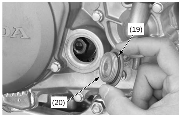
(19) junta tórica (20) tapa del orificio del cigüeñal
