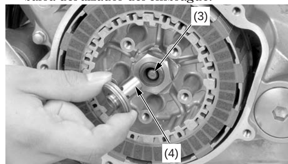
(3) barra del alzador del embrague (4) alzador del embrague
