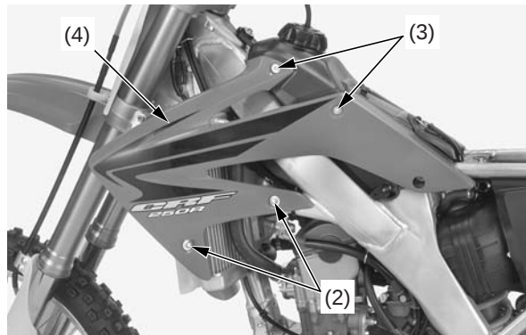
(2) pernos A/collares de los protectores (3) pernos B de los protectores (4) protectores
