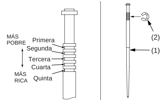
(1) sección recta
