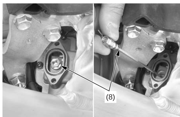
(8) conjunto de la aguja del surtidor/soporte
