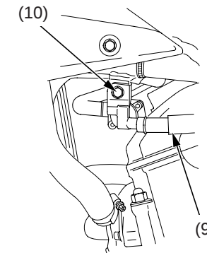
(9) línea de combustible (10) perno de la válvula del combustible
