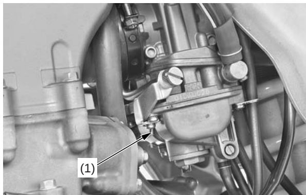
(1) tornillo piloto
