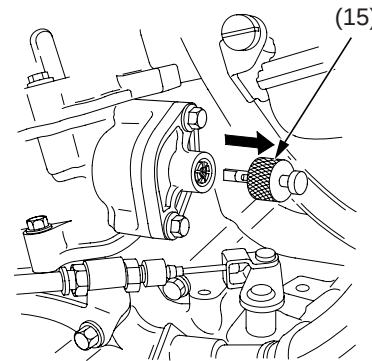
(15) tope del tensor
