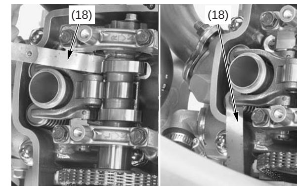
(18) calibre de espesores
