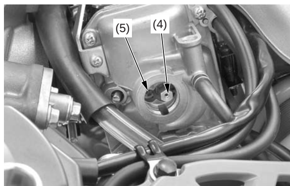
(4) surtidor principal (5) surtidor lento
