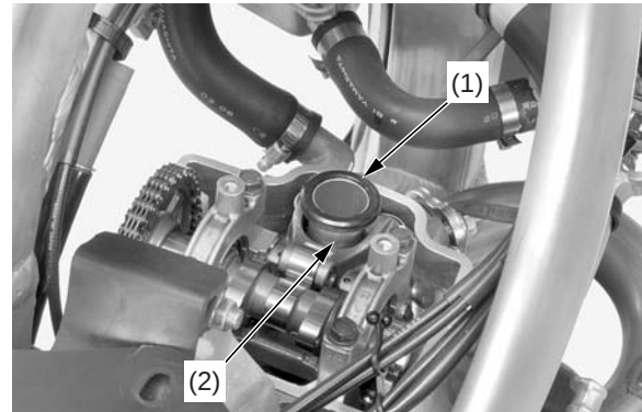
(1) empaquetadura del orificio de la bujía (2) orificio de la bujía
