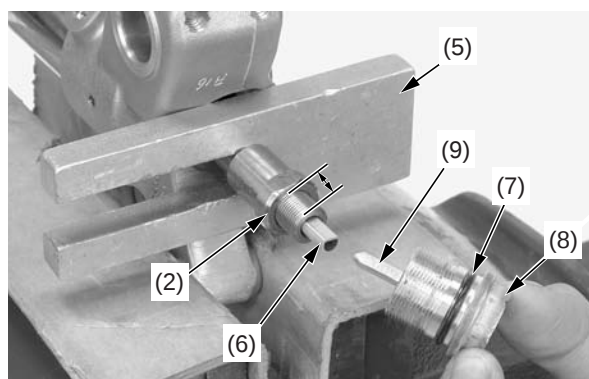
(2) contratuercas (7) Junta tórica (5) herramienta de tope (8) perno central (6) varilla de empuje (9) barra de ajuste
