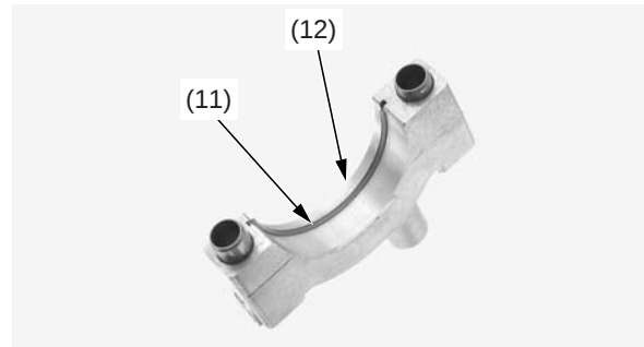
(11) anillo de ajuste (12) soporte del árbol de levas
